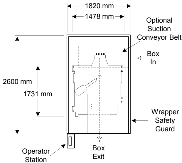
CMG-2000-W Wrapper
